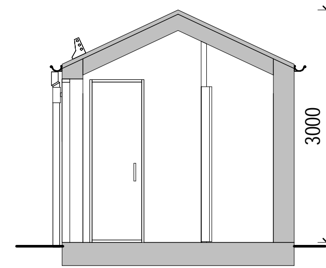
SEKTION A-A
